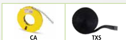
DFT
